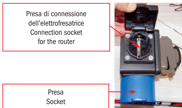
Figura 12 - Connessione elettrica
